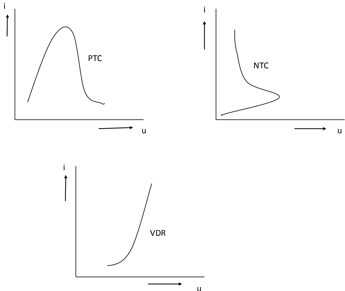
Àwòrán 1 : Àwọn ifidámọ̀ àwọn àtākò PTC, NTC àti VDR(I/U)
